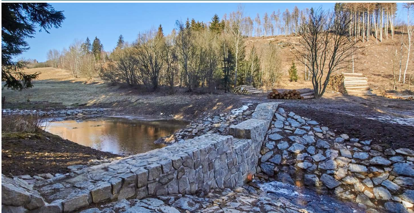
Dokončená vodní nádrž „Na koupeli“ v Hlubokém u Kunštátu.
